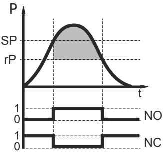
迟滞模式
