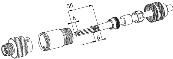
内部电缆连接 (螺钉连接) 4、5芯微螺钉连接
