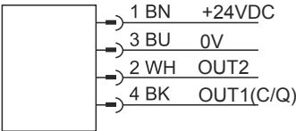
接线图
